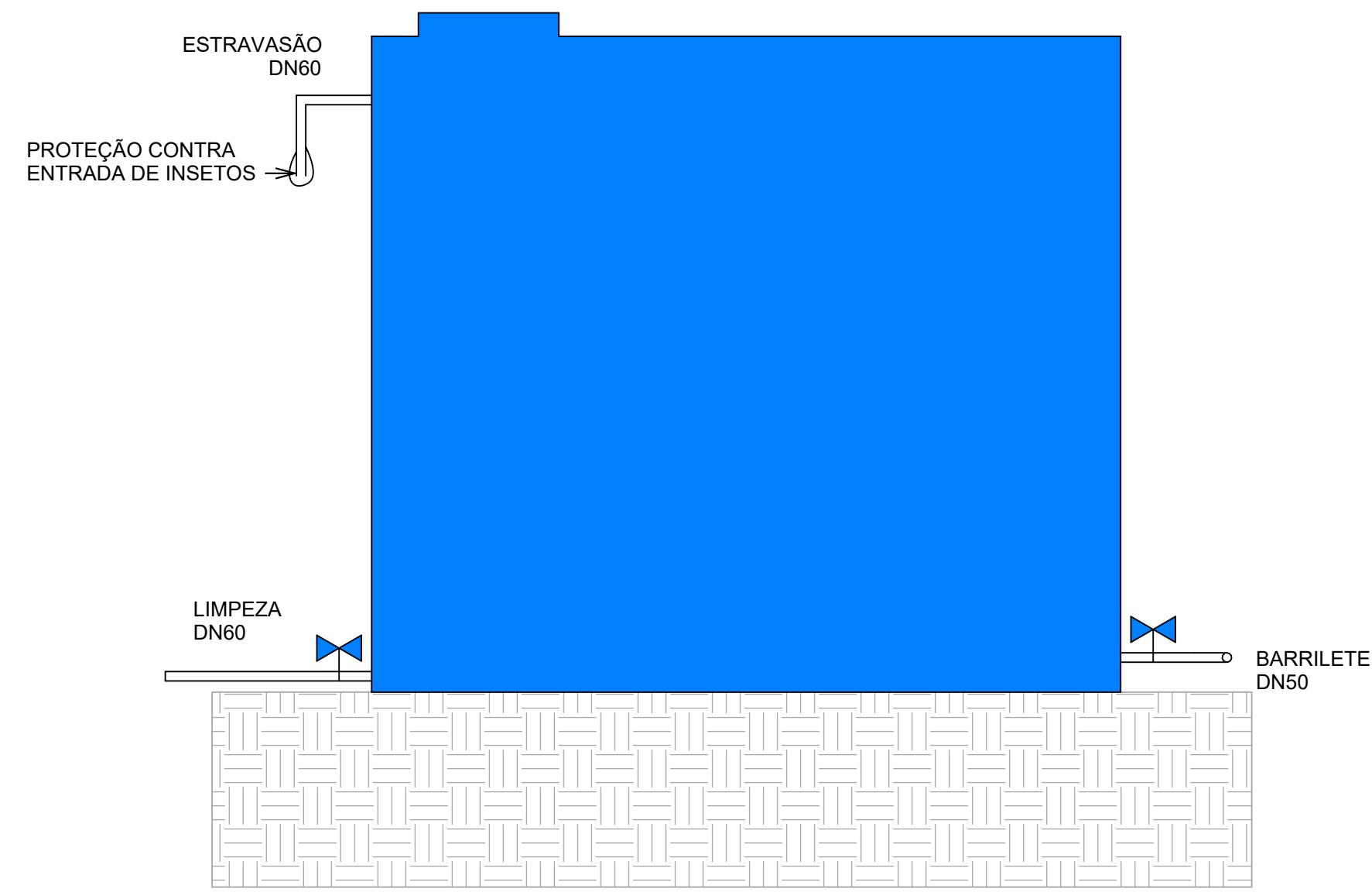
6 DET. ESTRAVASÃO/TUBO LIMPEZA 1 : 25
