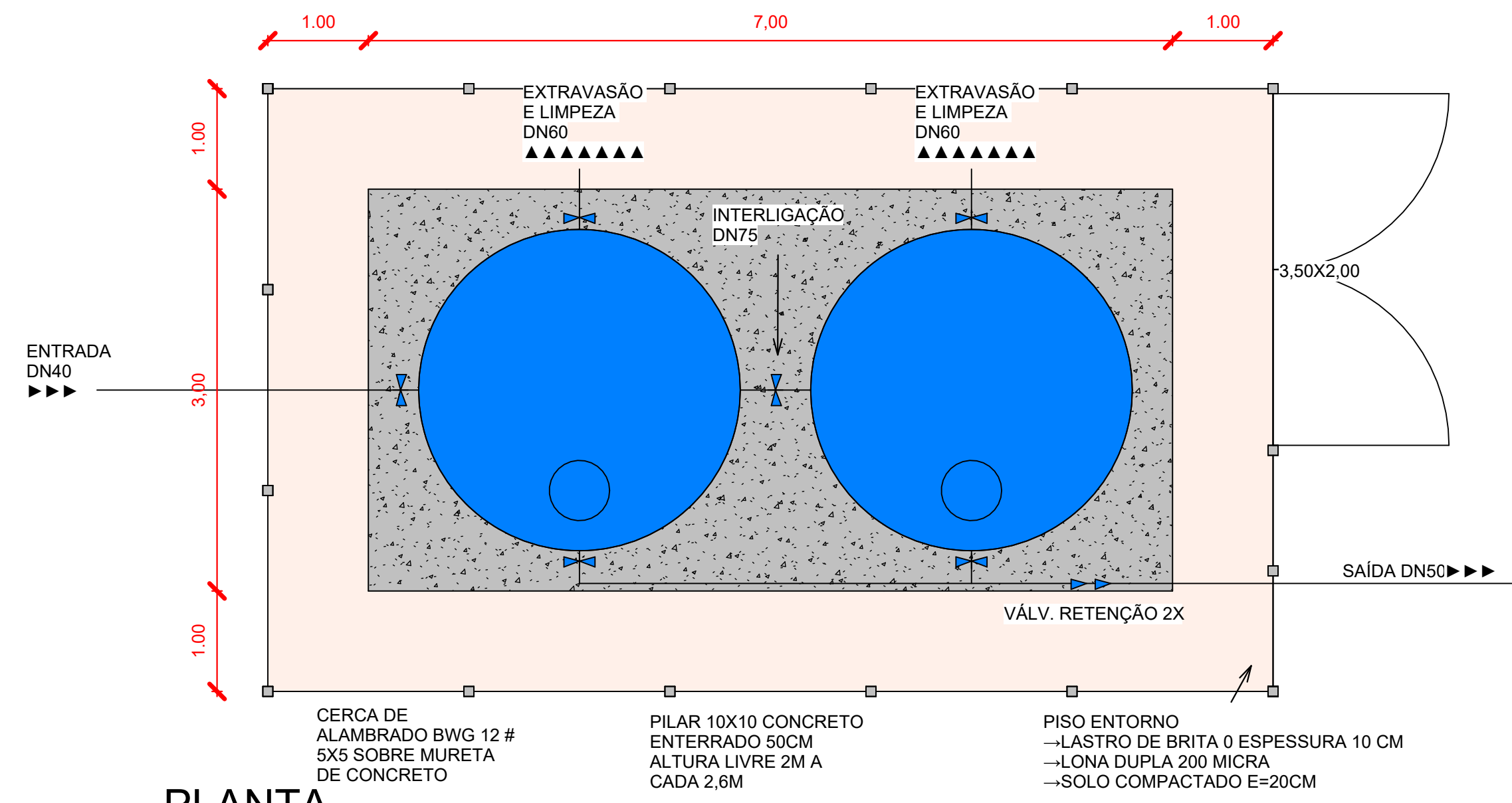
2 PLANTA RESERVATÓRIOS 1 : 50
