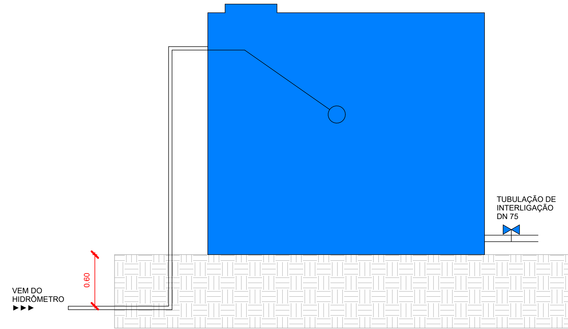
5 DET. RAMAL ALIMENTADOR 1 : 25
