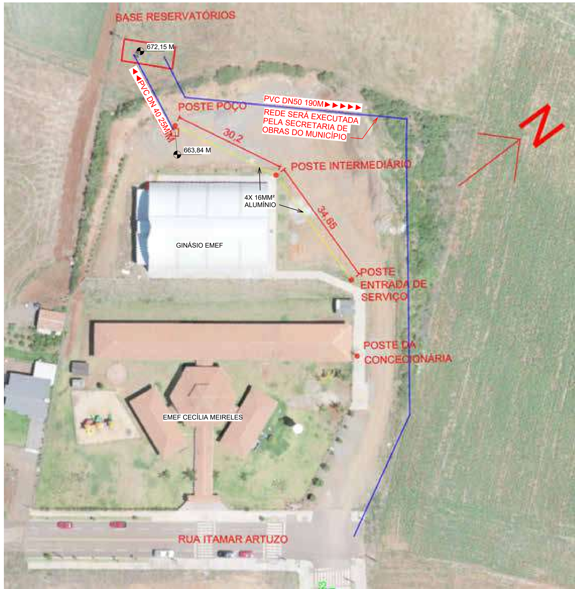
1 SITUAÇÃO 1 : 500
