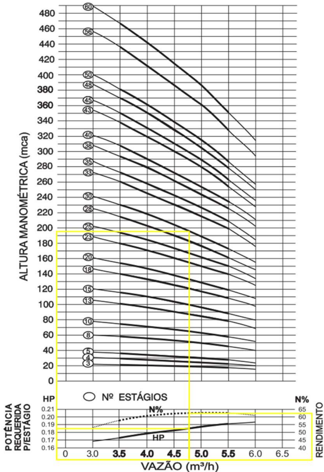
Figura 1: CURVA DA BOMBA VAMBRO VBOP44 (REFERÊNCIA)
